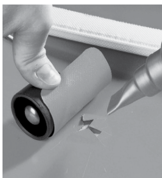
Aplicare plăsturi de sudură
