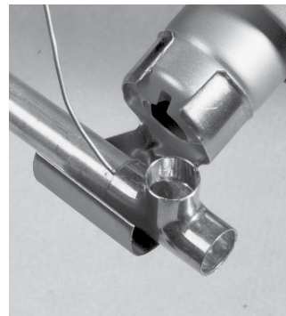
Lipire țevi cupru
