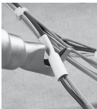
Contractare manșon izolant
